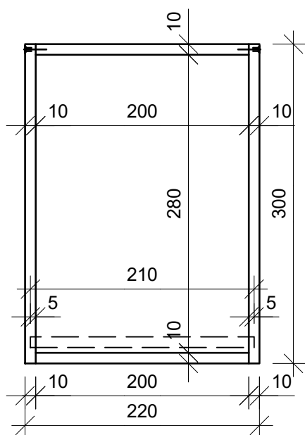
Schnitt A-A
