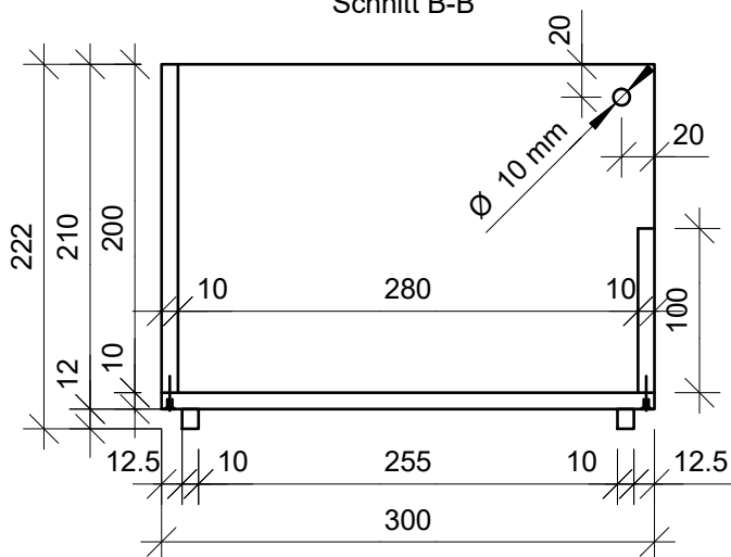
Schnitt B-B
